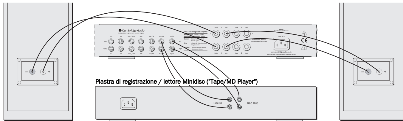
Amplificatore integrato Azur 65
