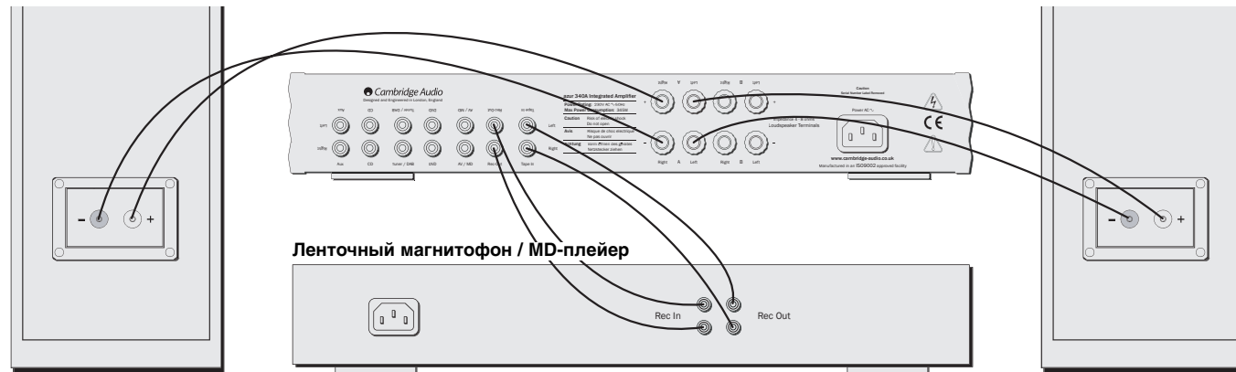
Комбинированный усилитель серии azur 107
