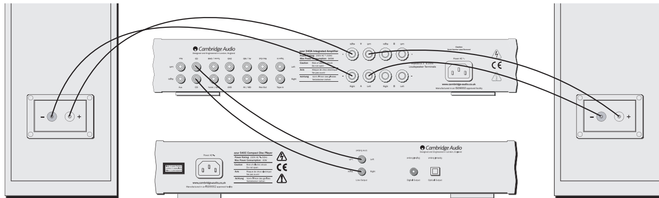
50 amplificador integrado azur
