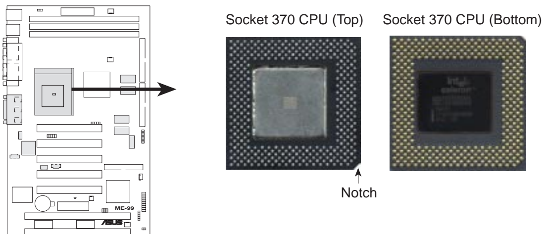
ME-99 Socket 370
