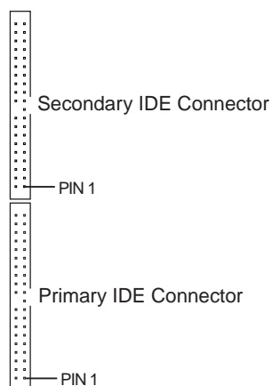
ME-99 IDE Connectors
