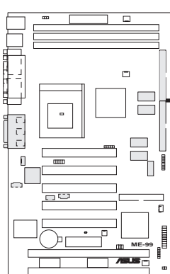
ME-99 IDE Connectors
