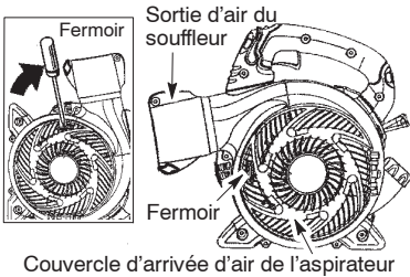
Couvercle d'arrivée d'air de l'aspirateur
